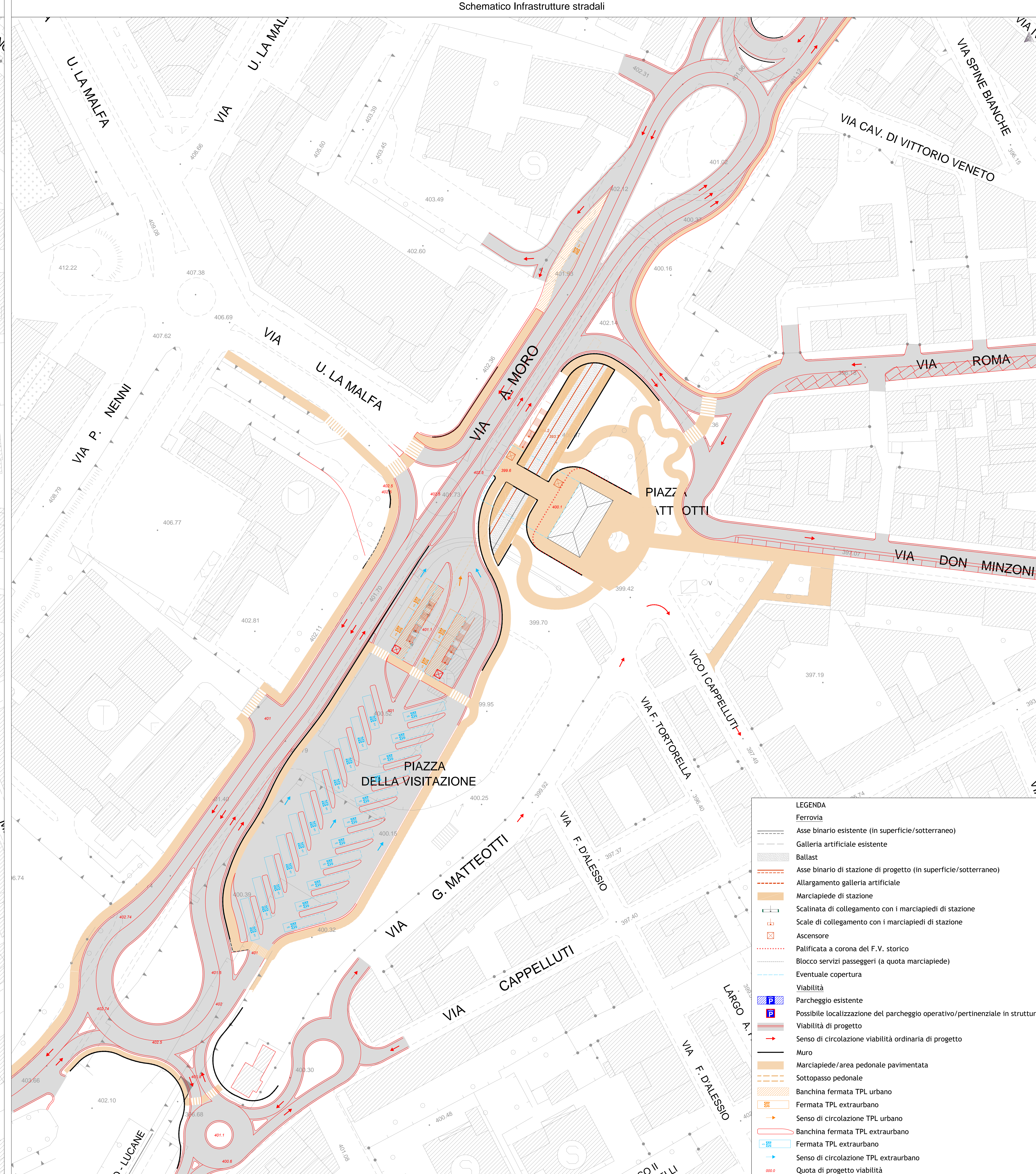
Schematico Infrastrutture stradali
