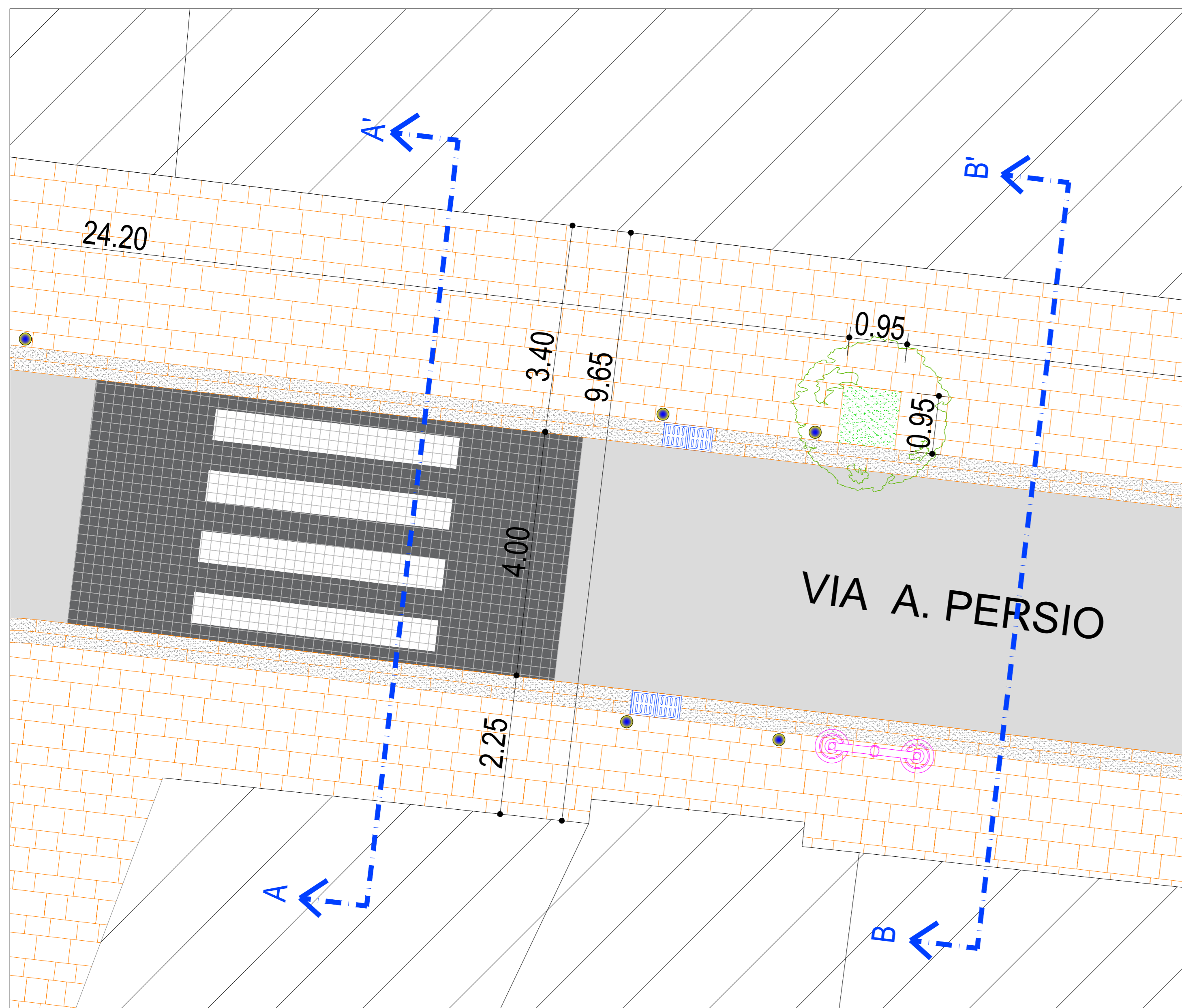
Pianta dettaglio scala 1:50
