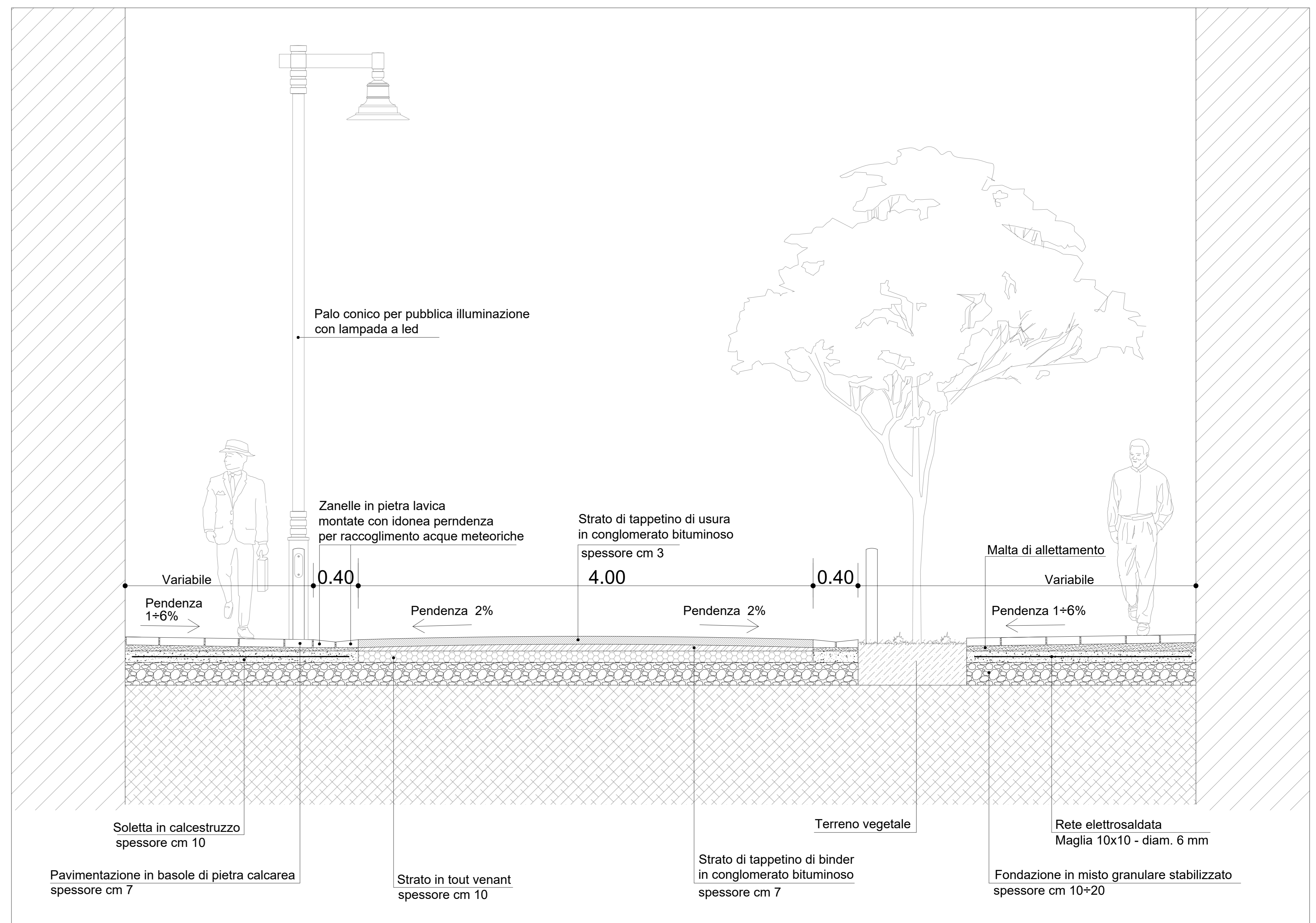
Sezione B-B' scala 1:20
