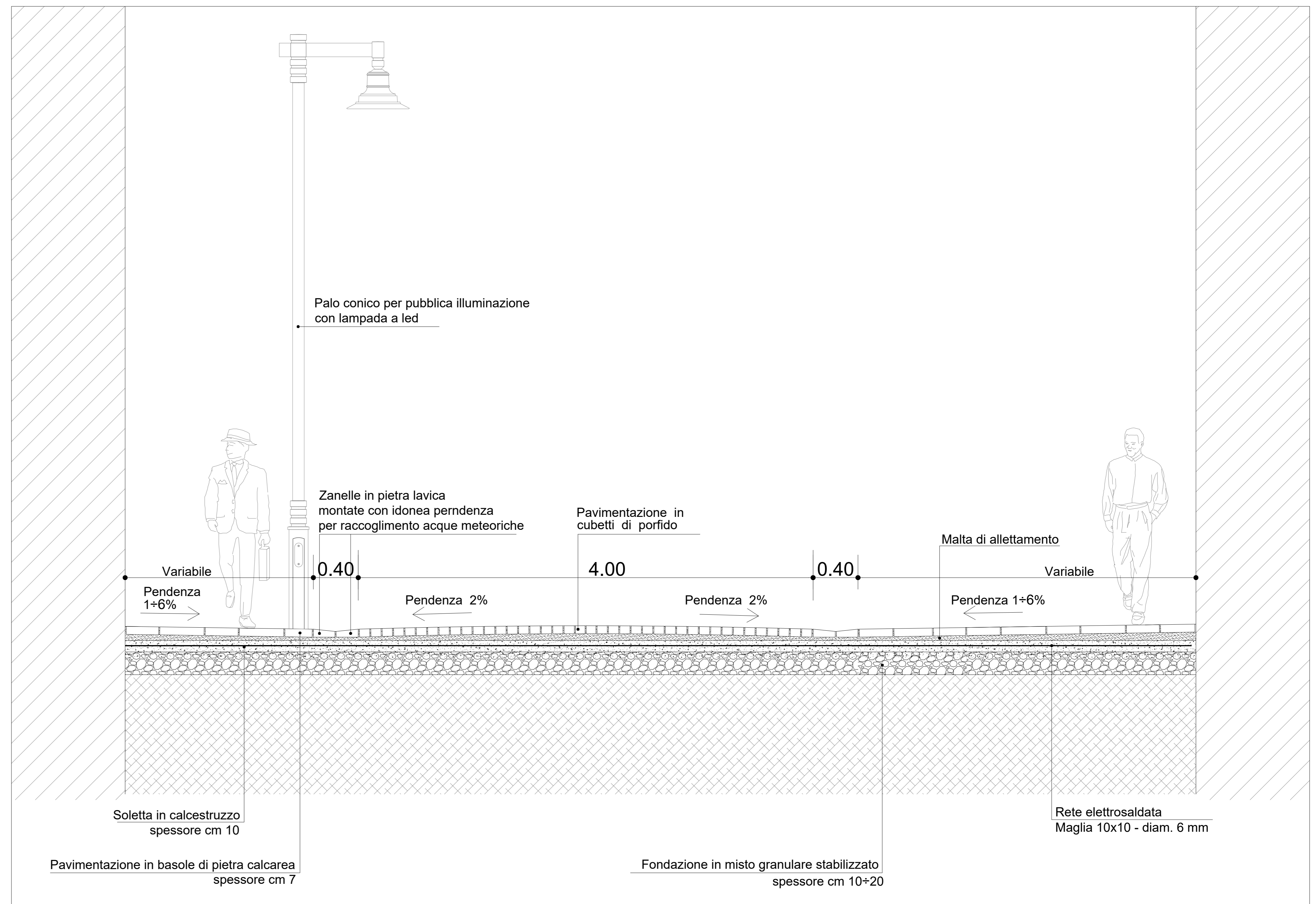
Sezione A-A' scala 1:20
